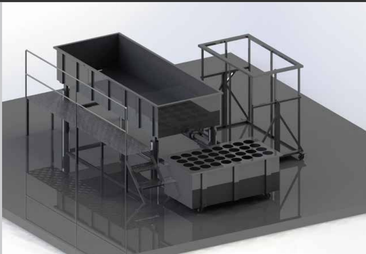
Planta para Fabricação de Frescal, Gorgonzola e Ricota
